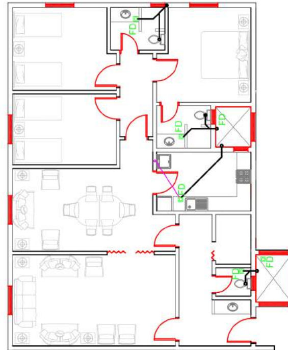
SEWERAGE SYSTEM مثال توزيع ماء تصريف المجاري داخل الشقة
