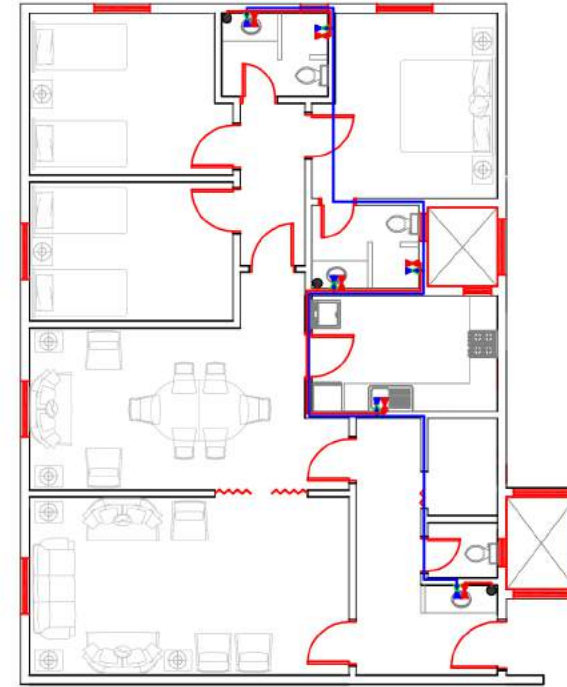
SWEET WATER مثال توزيع الماء الحلو داخل الشقة
