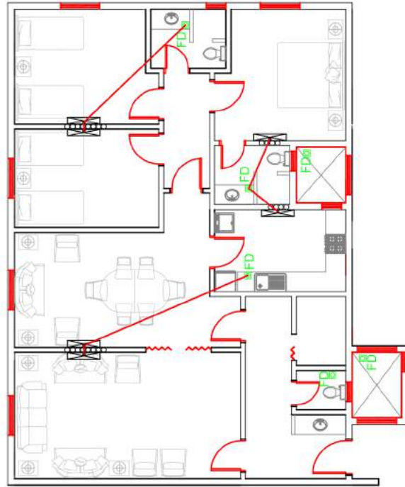
AIRCON DRAIN مثال توزيع تصريف ماء المكيفات
